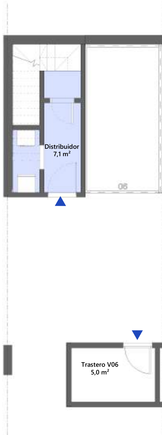
PLANTA SOTANO
