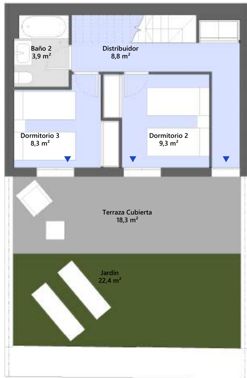
PLANTA SOTANO
