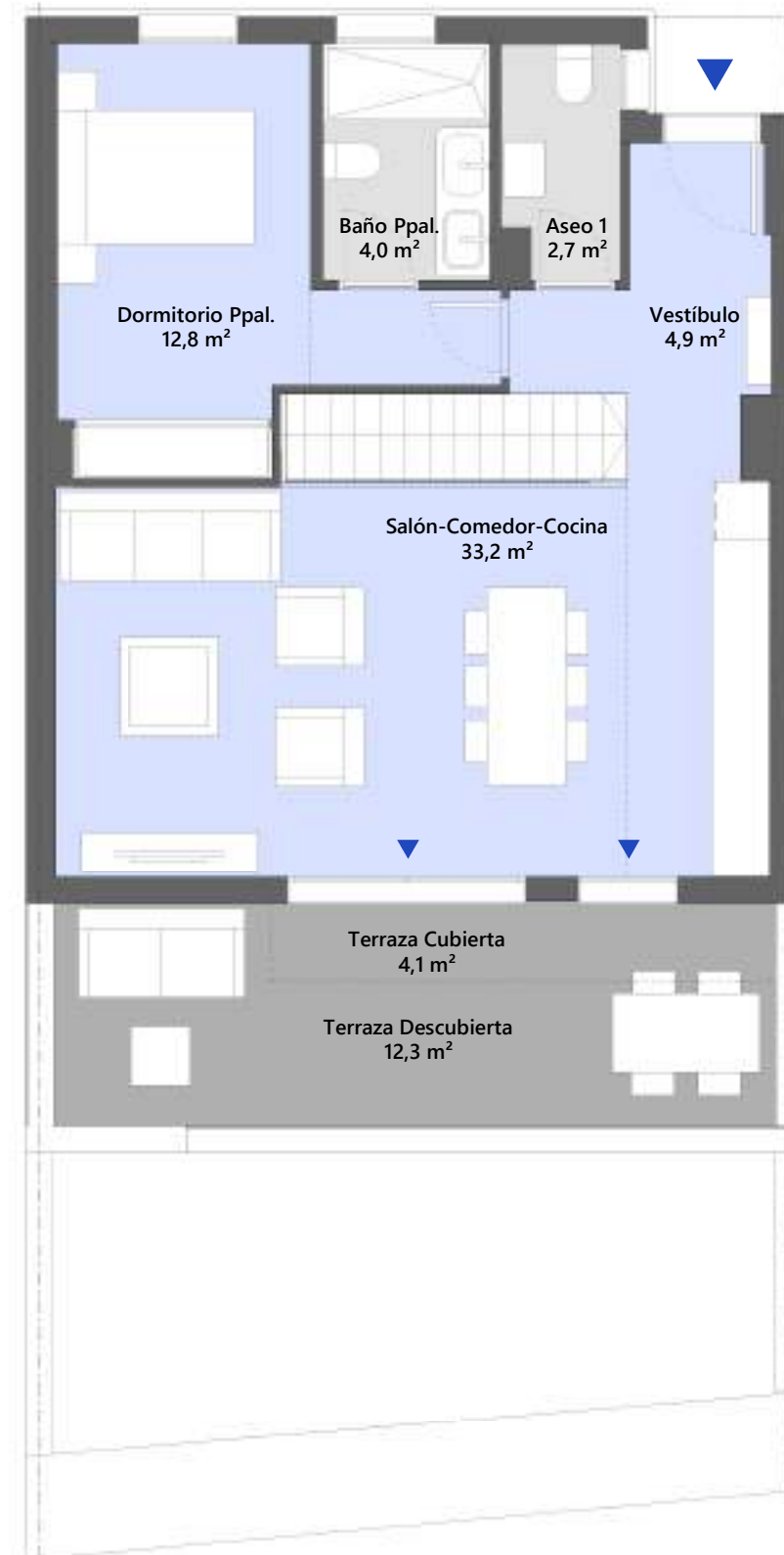
PLANTA BAJA
