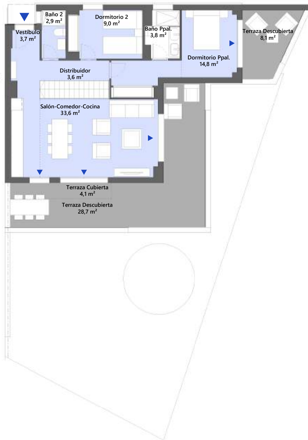
PLANTA BAJA
