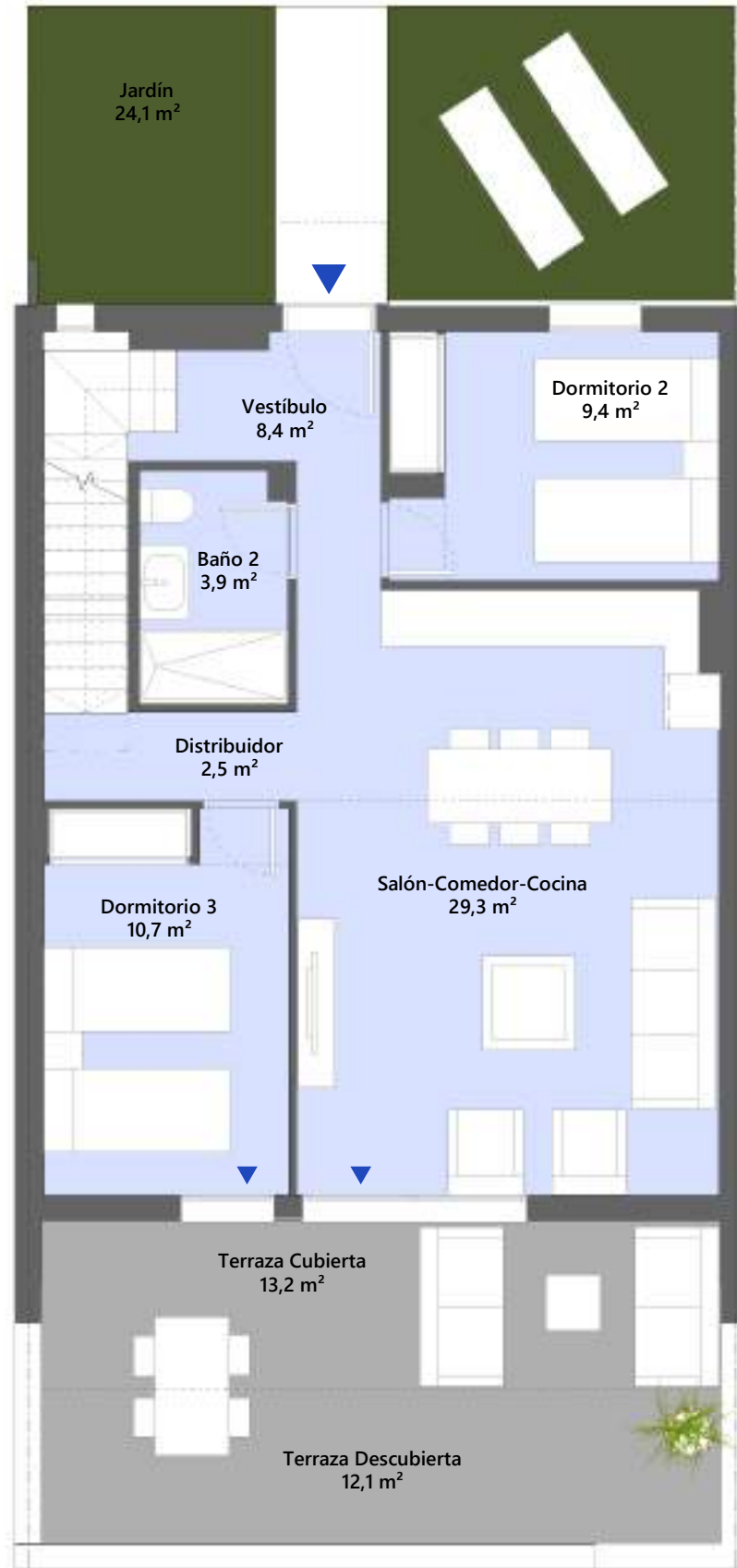
PLANTA BAJA
