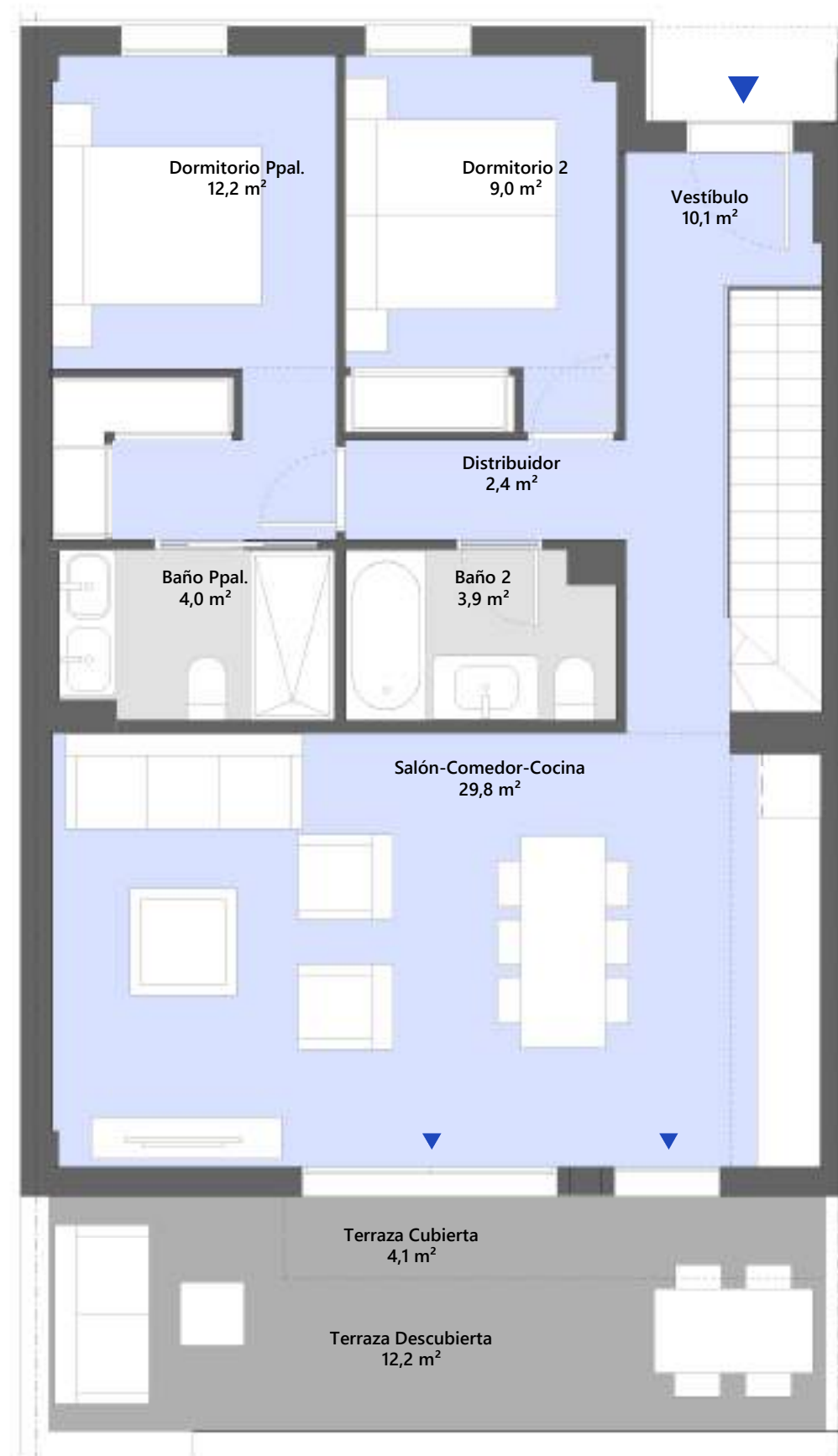
PLANTA BAJA
