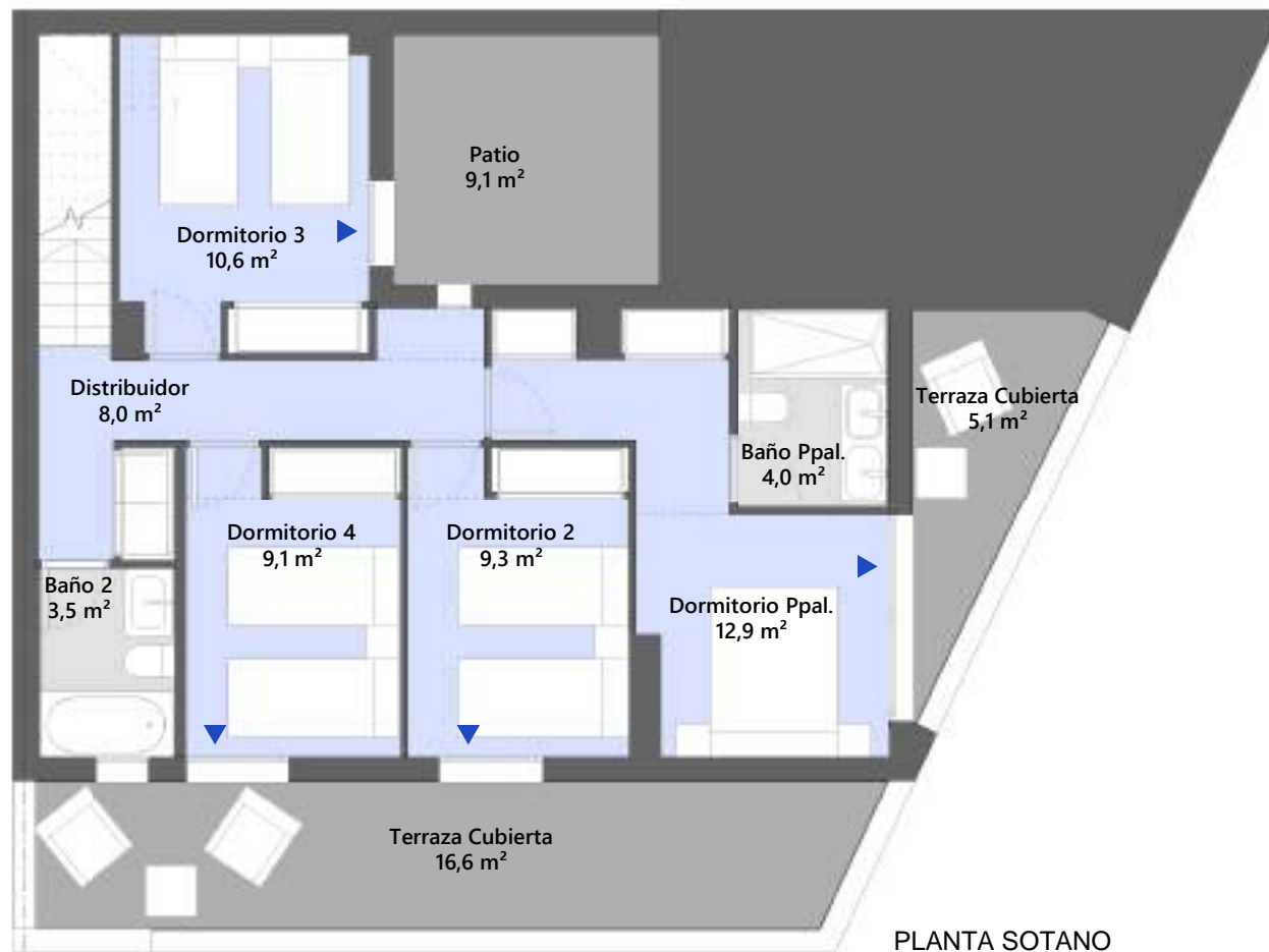
PLANTA SOTANO
