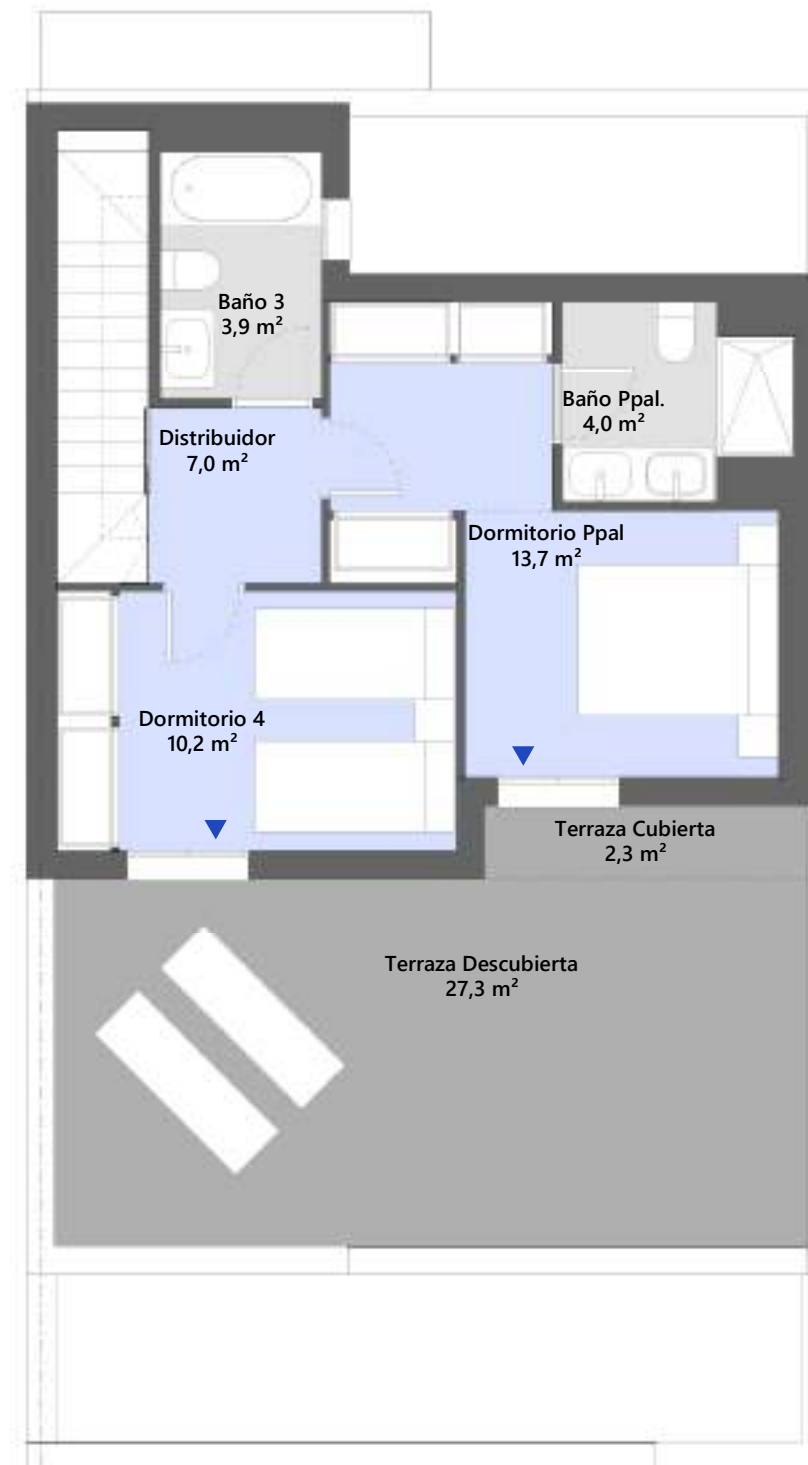
PLANTA PRIMERA
