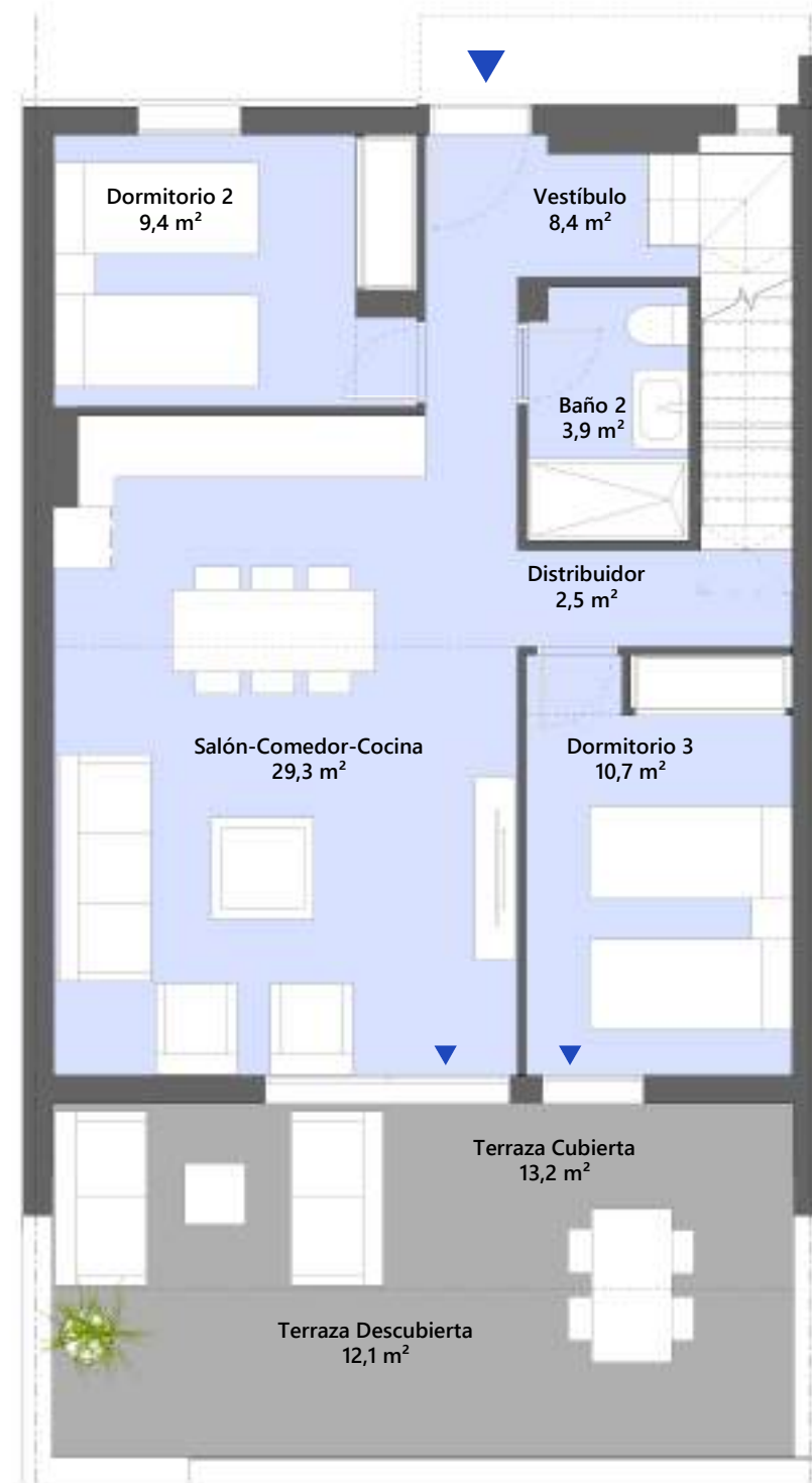
PLANTA BAJA
