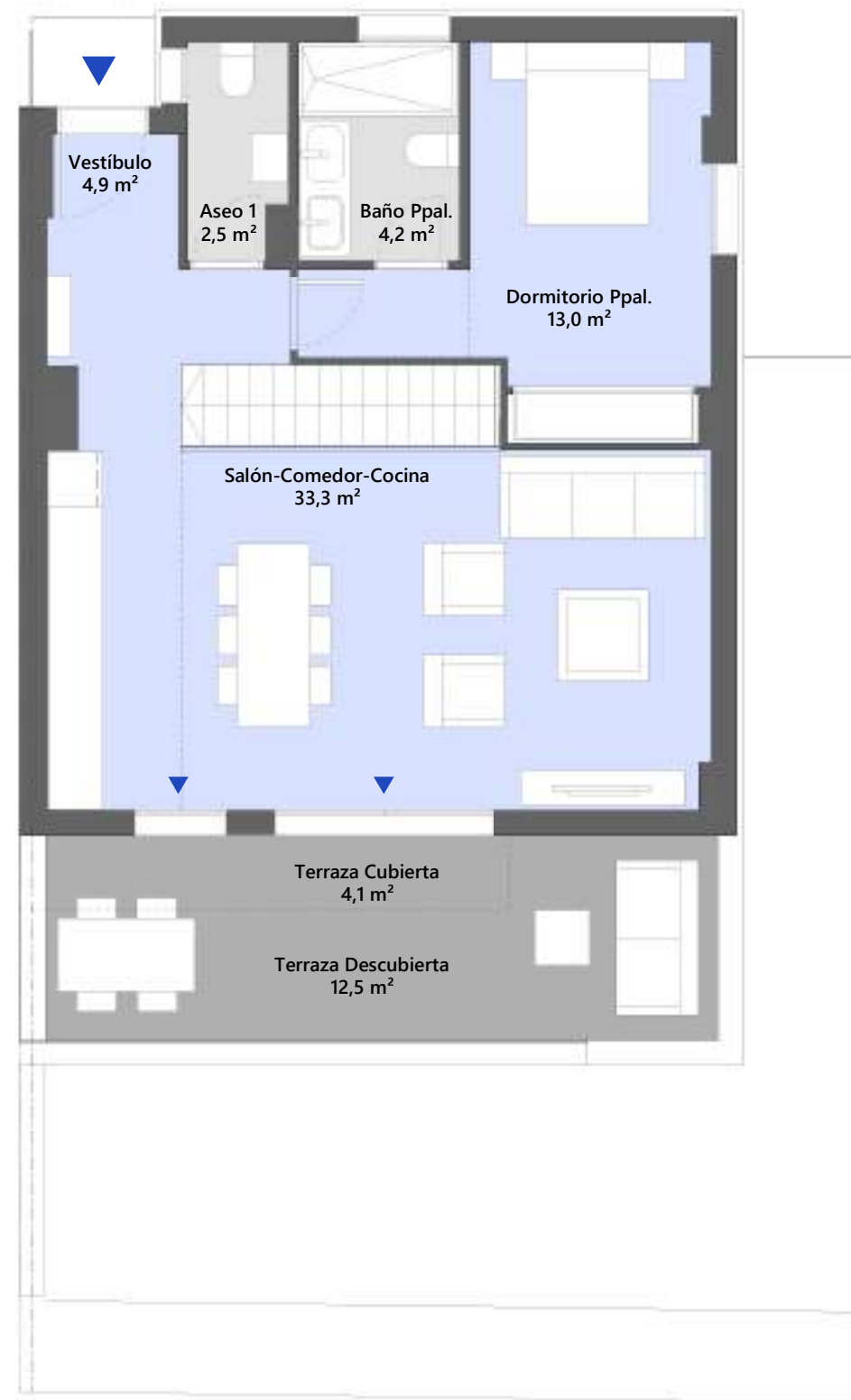
PLANTA BAJA
