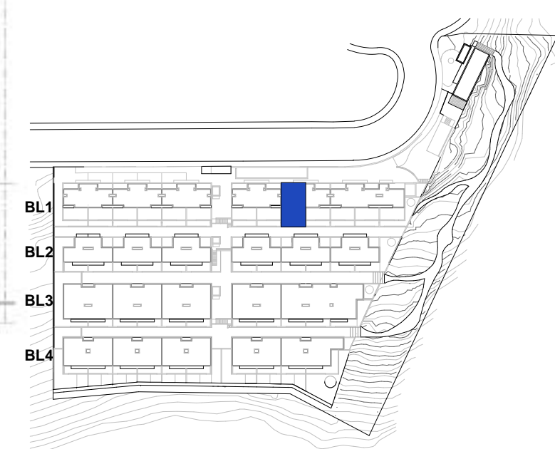
Planta Cubierta
