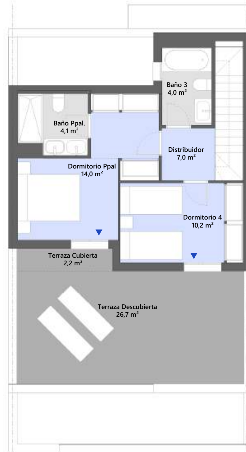
PLANTA PRIMERA
