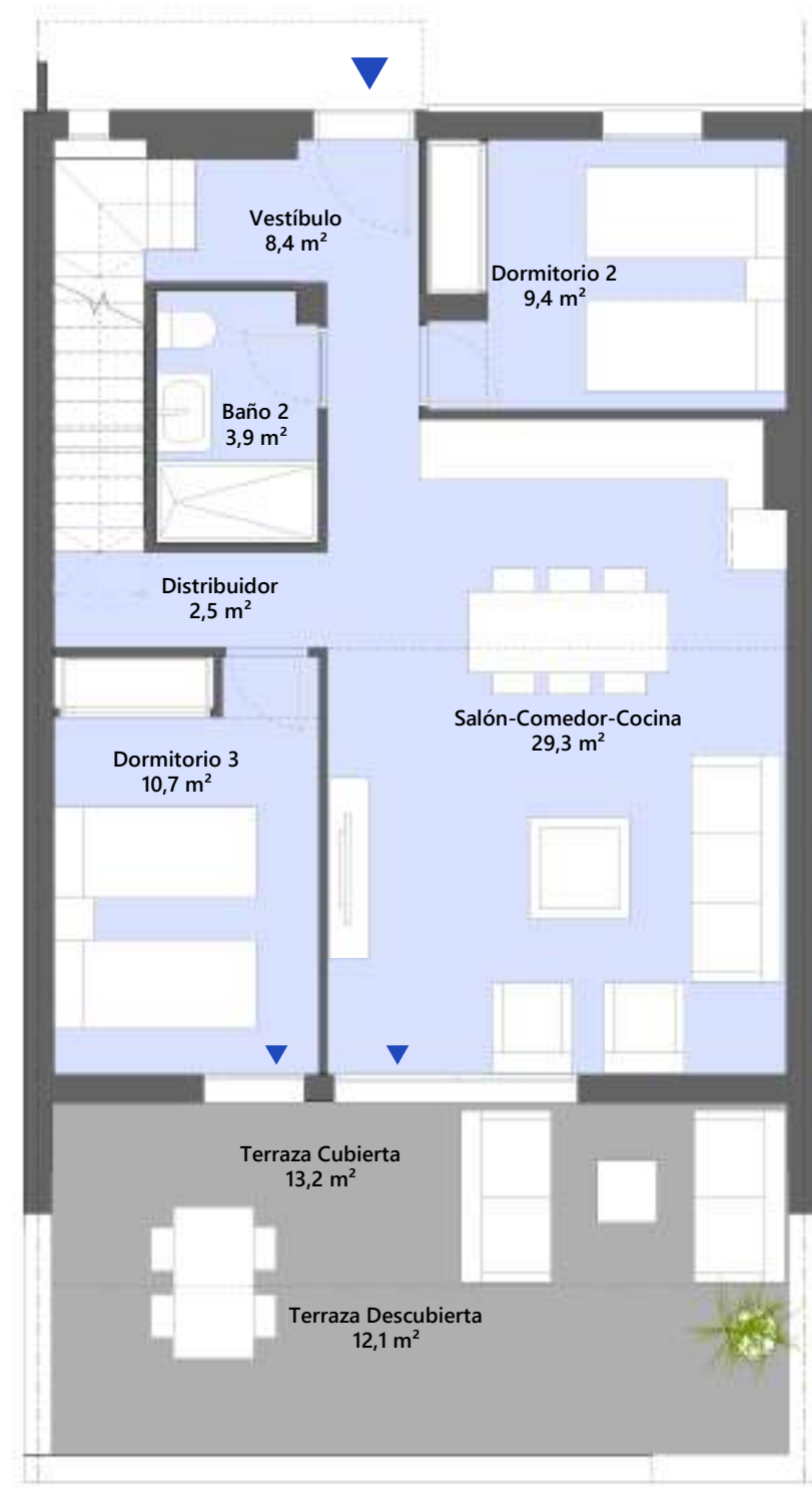
PLANTA BAJA
