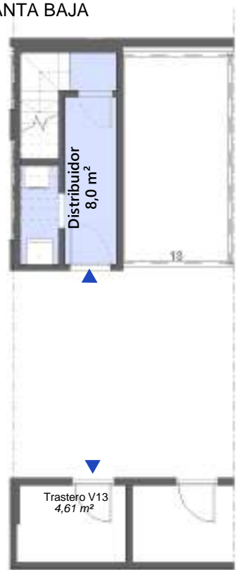
PLANTA SOTANO
